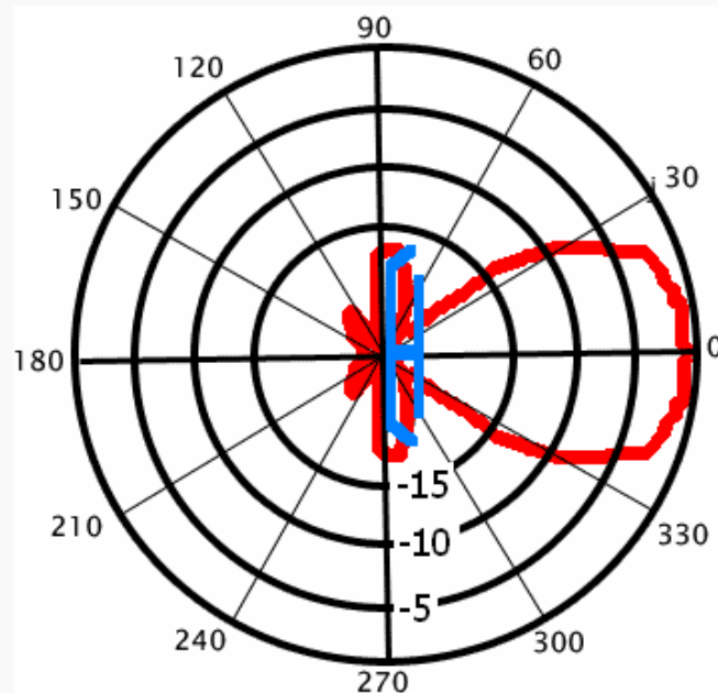
Типовая диаграмма направленности зигзагообразной антенны в горизонтальной плоскости
