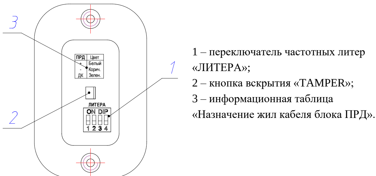
Рисунок 1.8 – Органы настройки блока ПРД извещателей «ФОРТЕЗА» (исполнение «bluetooth»)
