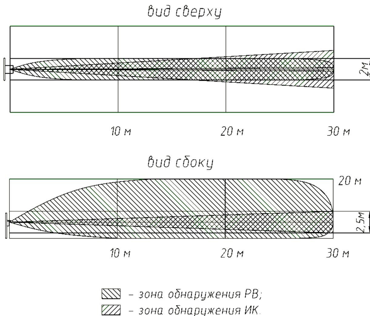
Рисунок 3.1 – Размеры зоны обнаружения извещателя «Циклоп-30»
