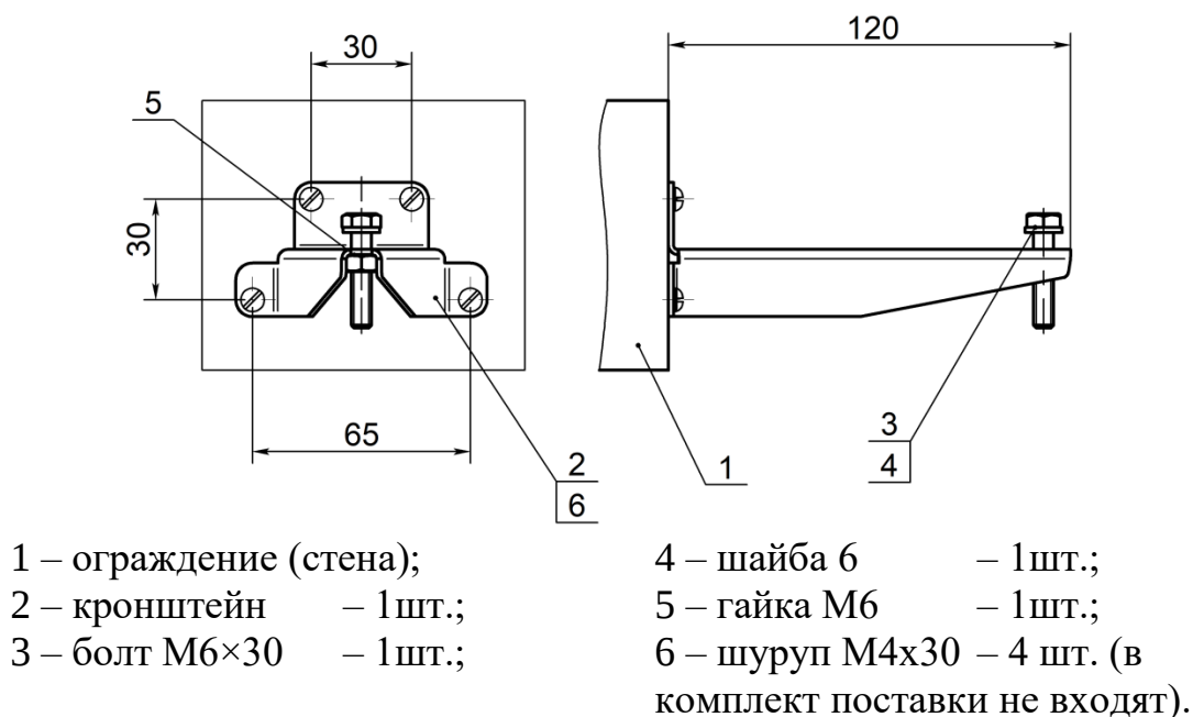
Рисунок 6.2 – Кронштейн с выносом 120 мм для установки извещателя на стену.
