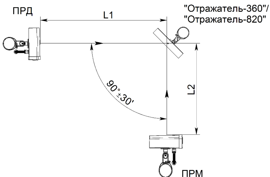
Рисунок 2.13 – Установка извещателей с применением отражателя «Отражатель-360» («Отражатель-820»)
