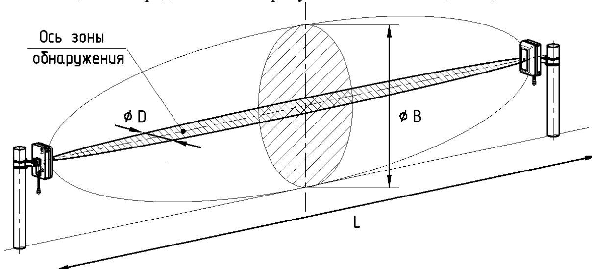
Рисунок 1.1 – Конфигурация зоны обнаружения
