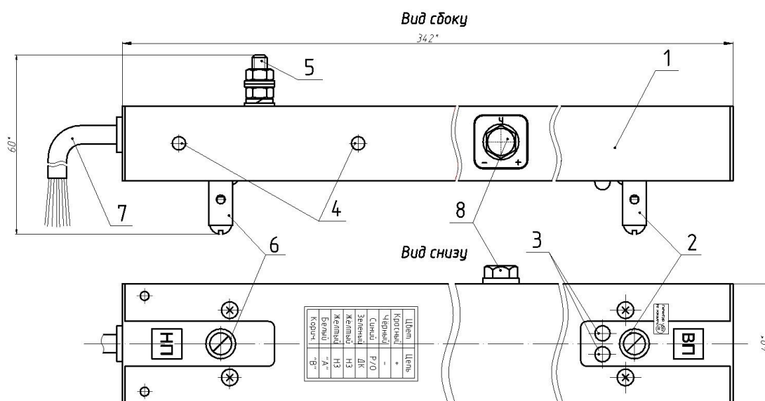
Рисунок 1.3 – Конструкция ПРМ.
