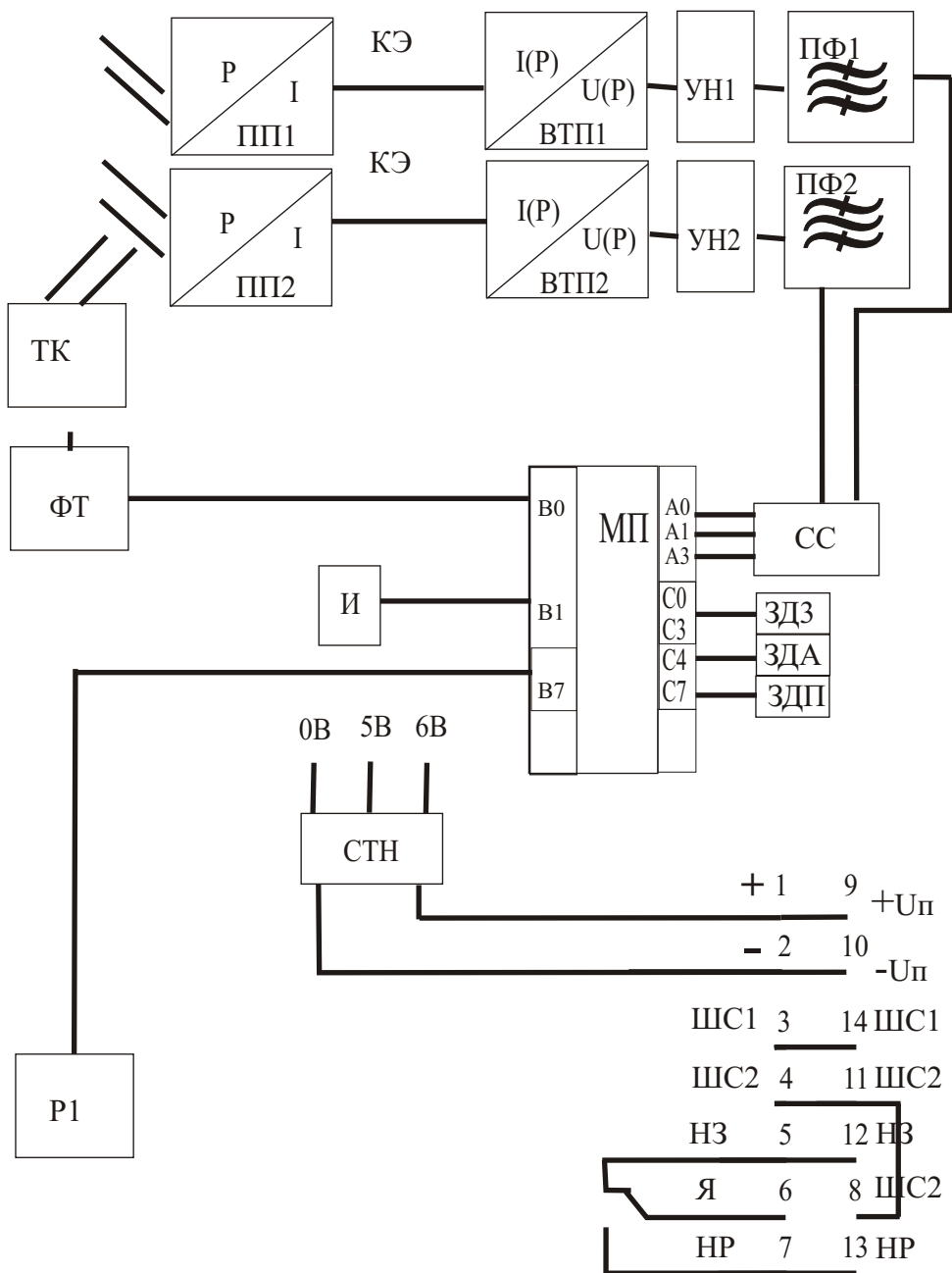
Рис3. Схема функциональная извещателя "Пульсар3-014СК"
