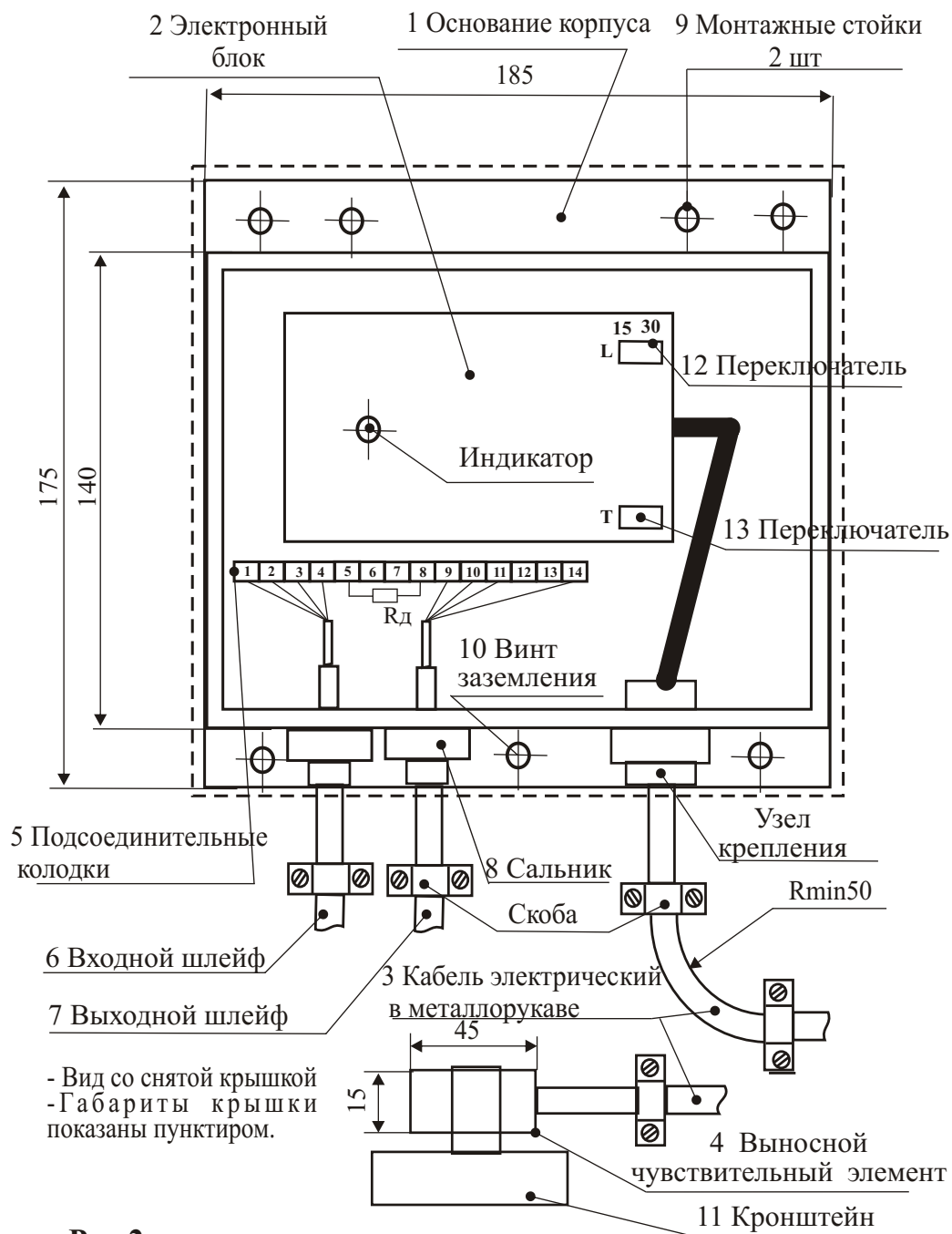
Рис 2 Извещатель “Пulsar4-011П”
