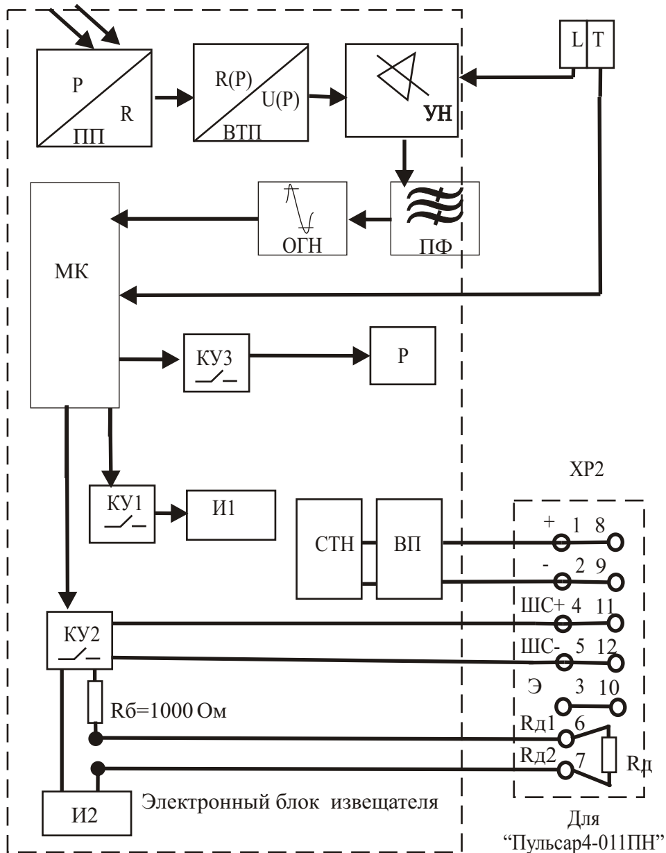
Рис 3 Схема функциональная
