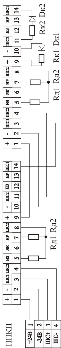
Рис. 6а Монтажная схема параллельного подключения “Пульсар4-013НК”, “Пульсар4-013СК”
