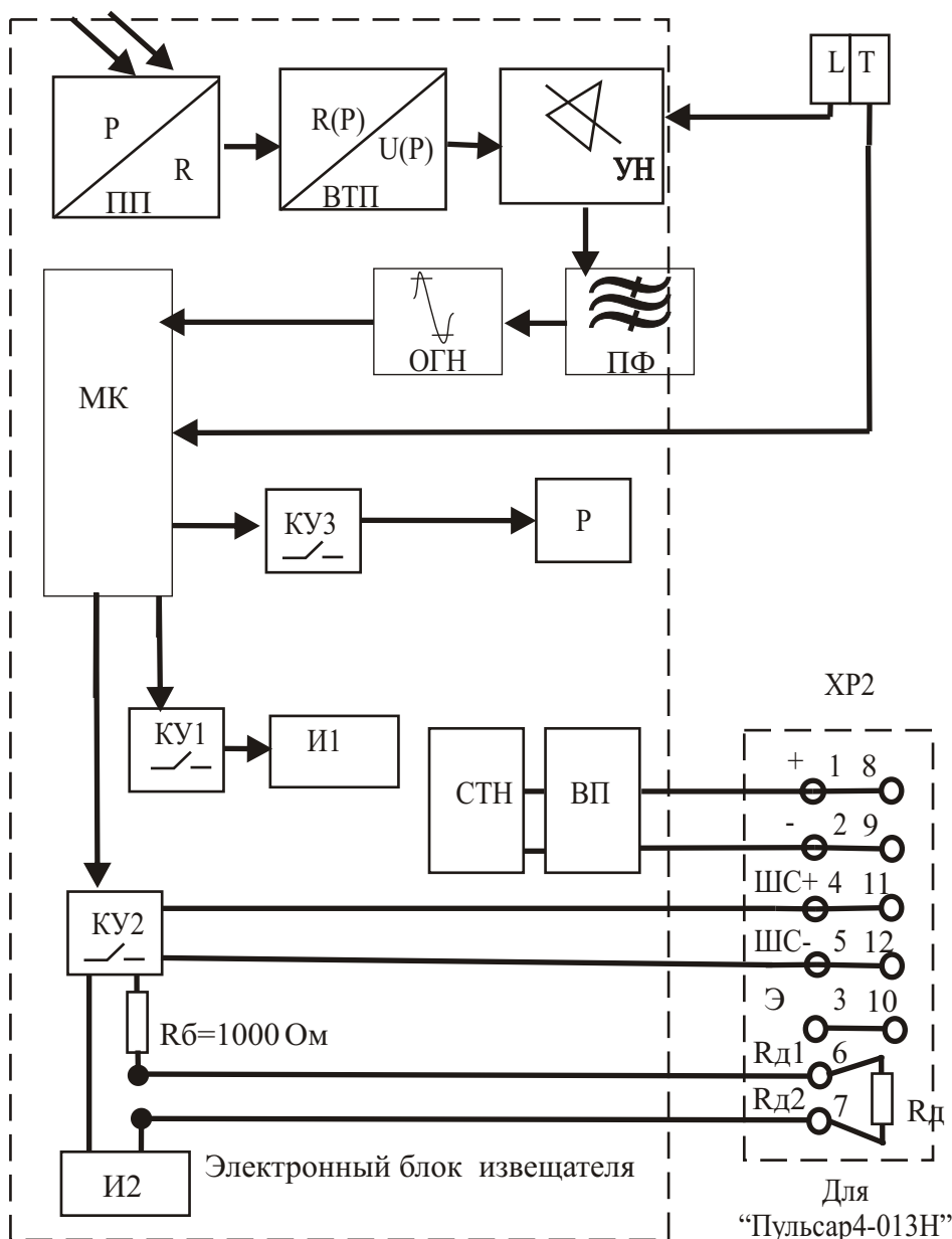
Рис 3 Схема функциональная
