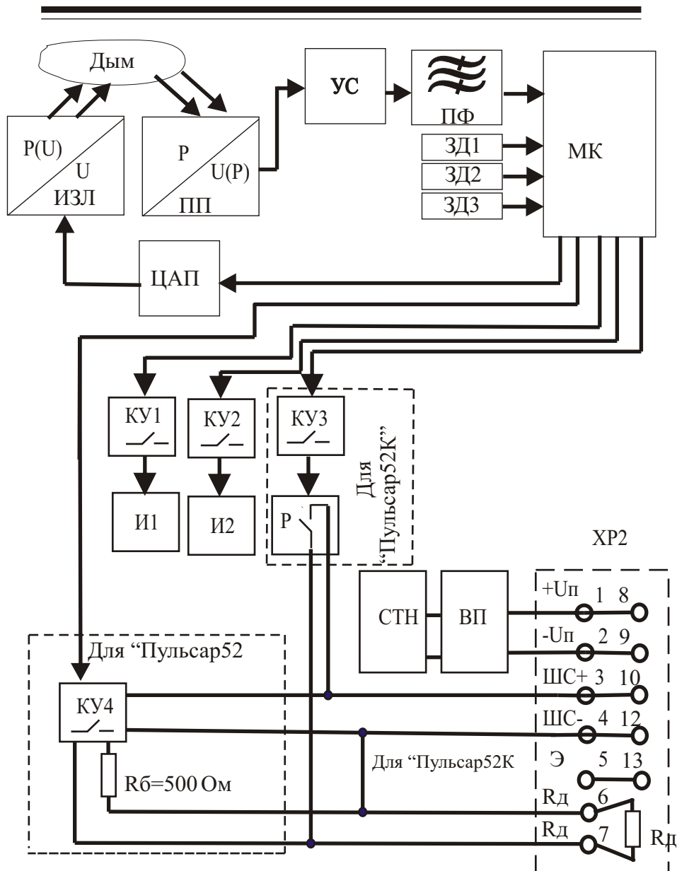
Рис. 1. Схема функциональная извещателя "Пульсар 52(В,Д)", "Пульсар 52К(В,Д)".
