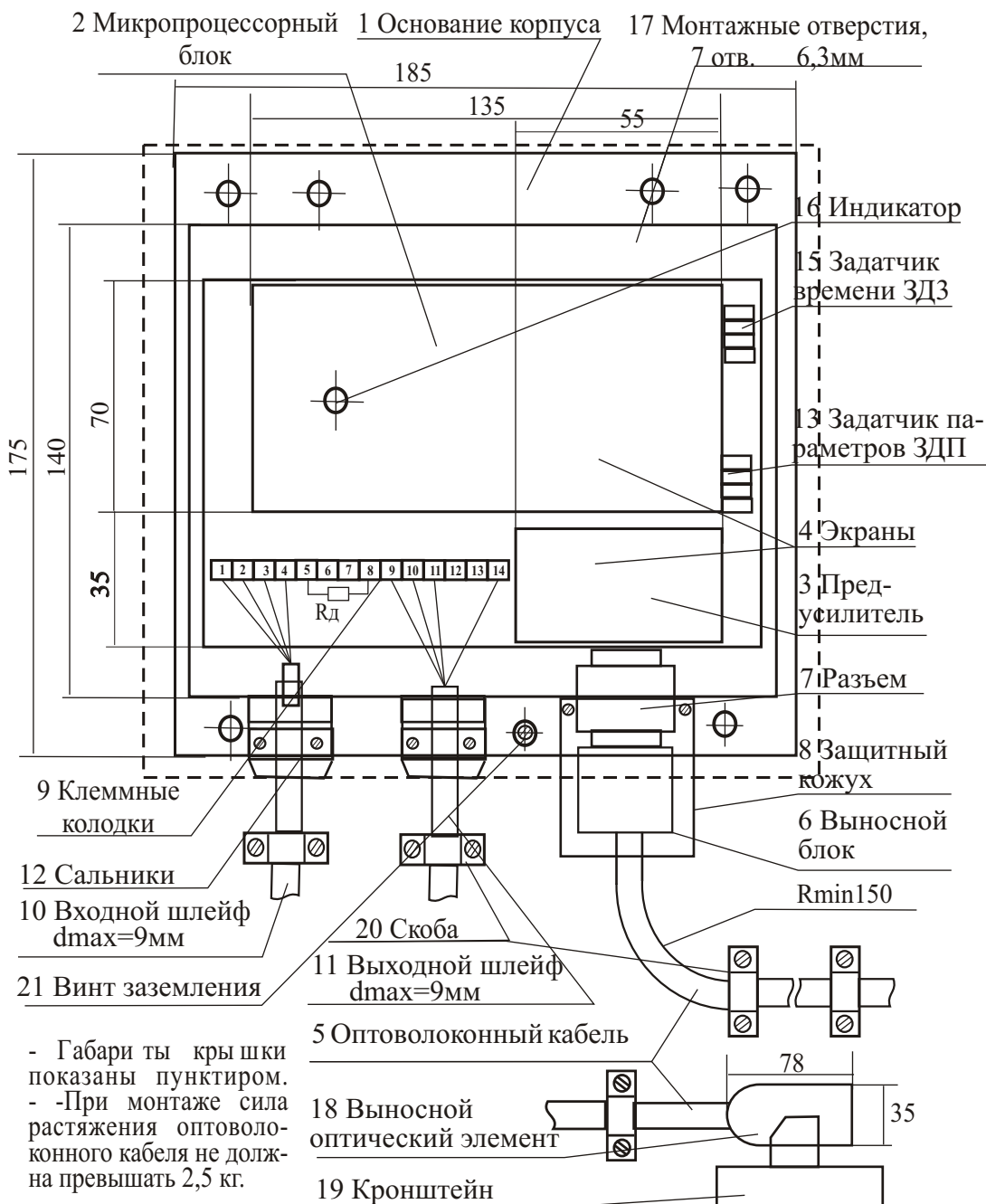
Рис 2а Извещатель пожарный пламени “Пульсар3-015К” вид со снятыми крышкой и защитной пластиной
