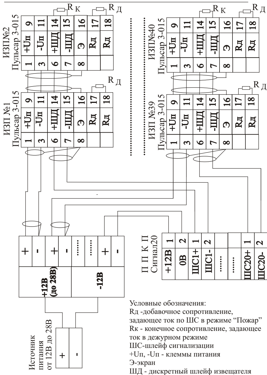
Рис. 5 Схема подключения извещателей “Пульсар3-015Н” “Пульсар3-015С” на примере ППКП “Сигнал20”
