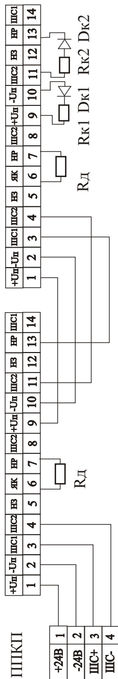
Рис. 8а Монтажная схема последовательного подключения “Пульсар3-014НК”, “Пульсар3-014СК” С нормально разомкнутым контактом реле
