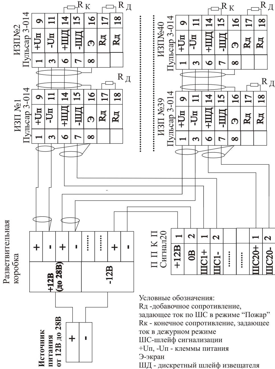
Рис. 5 Схема подключения извещателей "Пульсар3-014Н" "Пульсар3-014С" на примере ППКП "Сигнал20"
