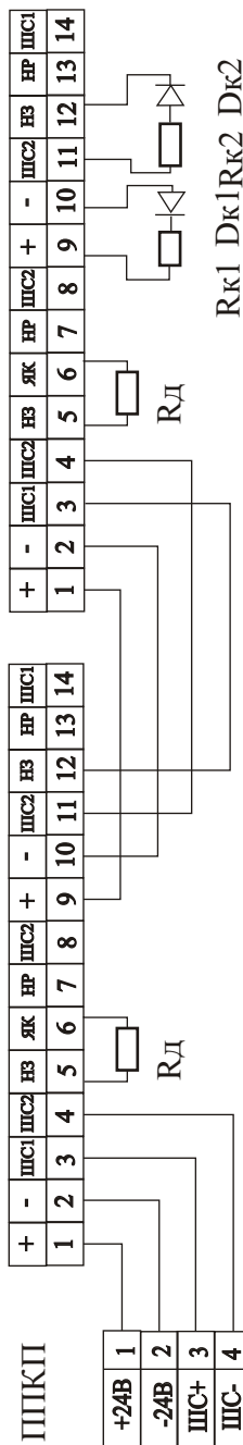
Рис. 7а Монтажная схема последовательного подключения “Пульсар4-013НК”, “Пульсар4-013СК” с нормально замкнутым контактом реле
