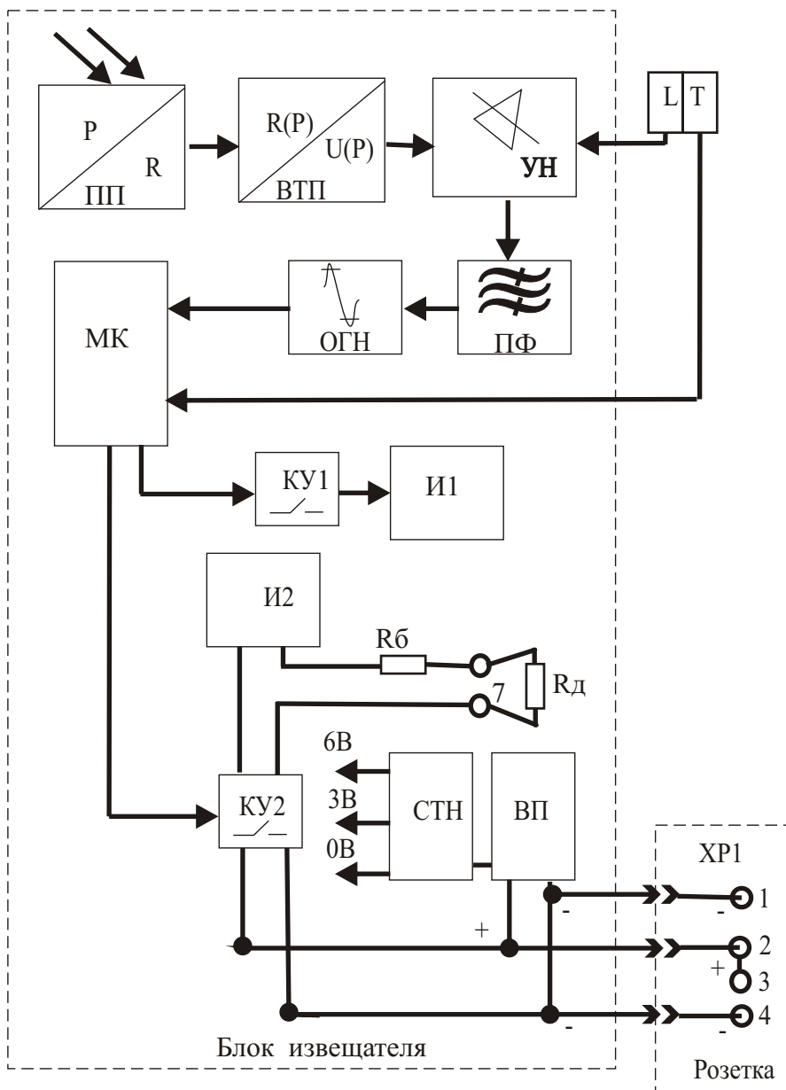
Рис 7 Схема функциональная
