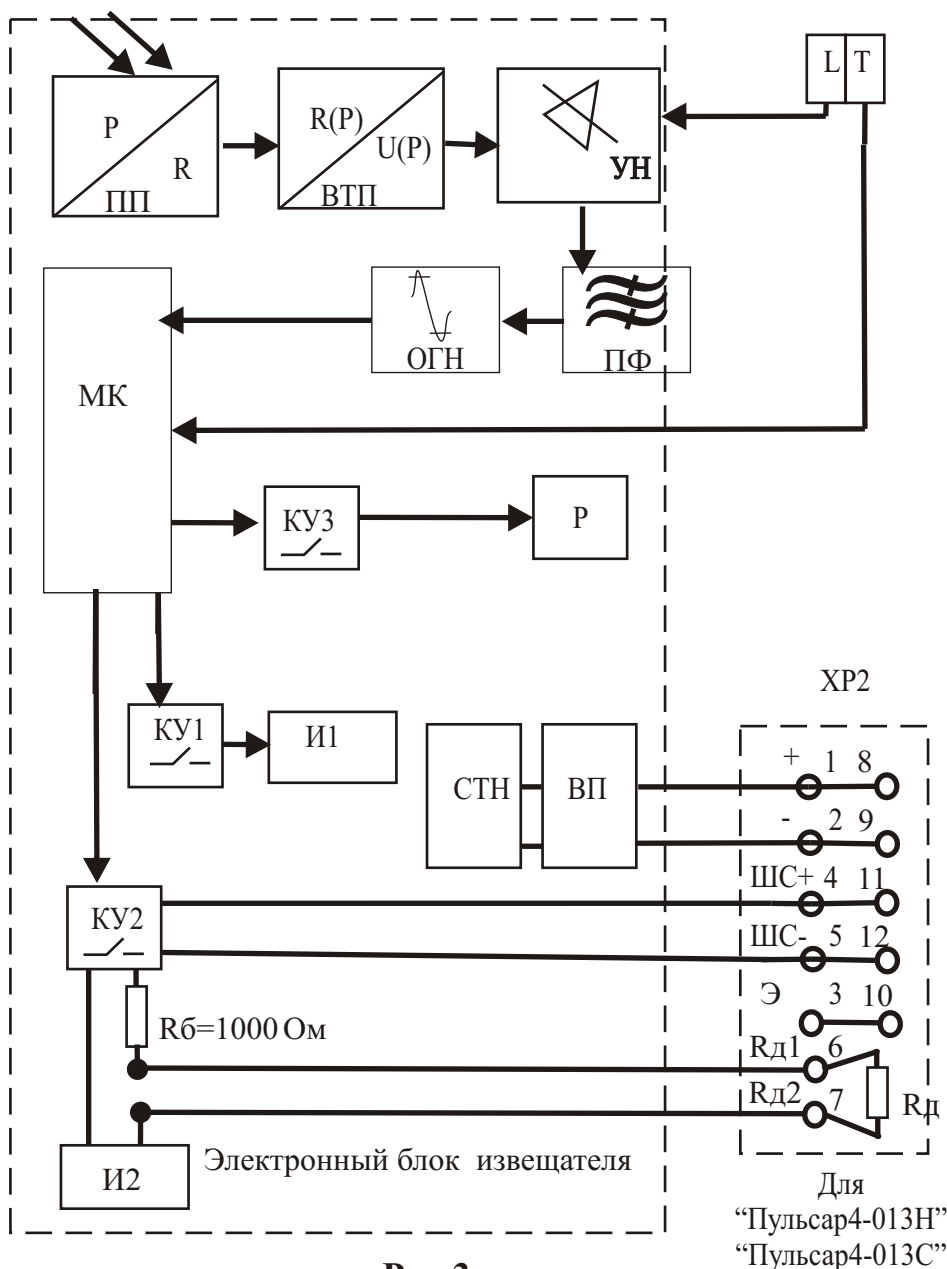
Рис 3 Схема функциональная
