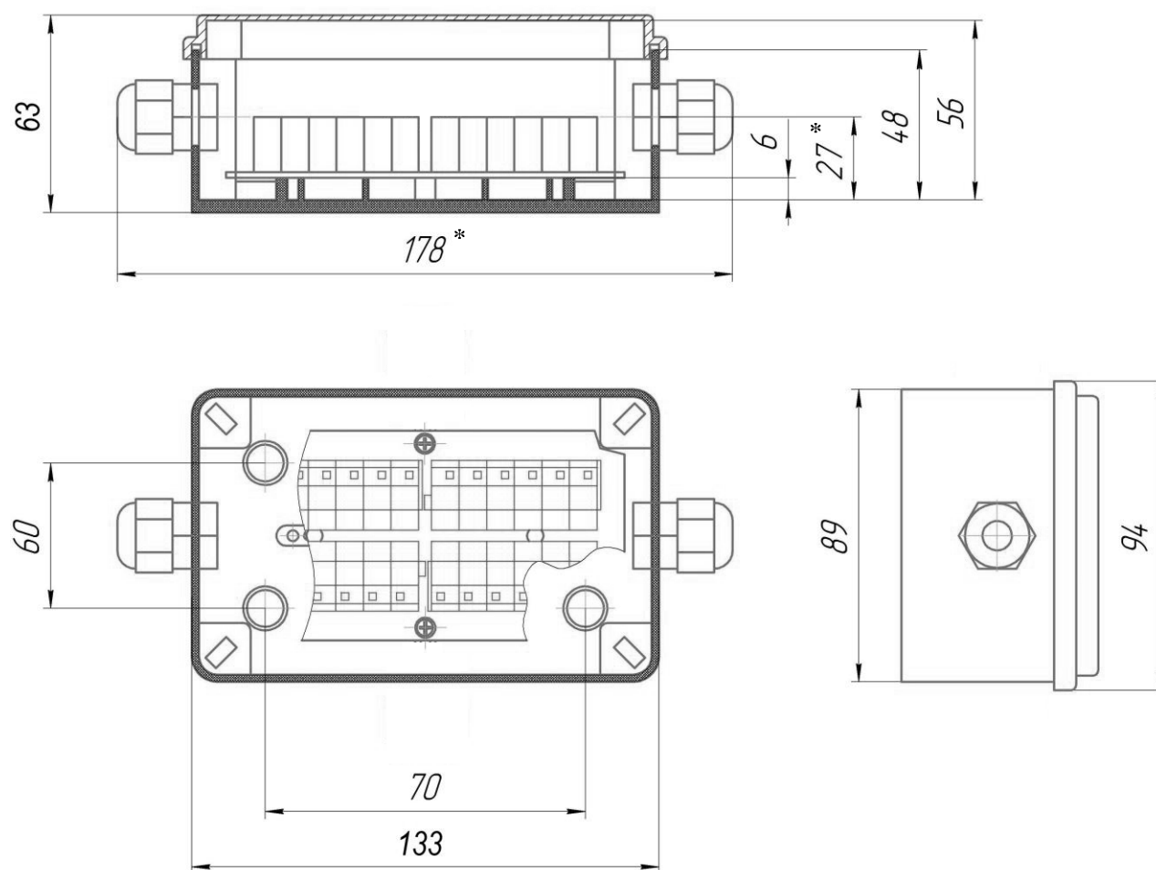
Рисунок А1. Установочные размеры коммутационной коробки извещателя.
