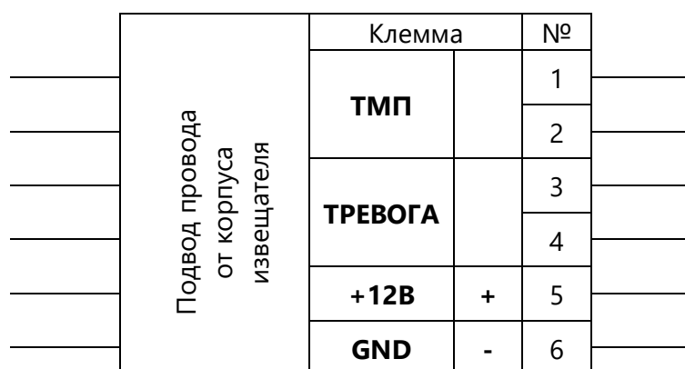
Рисунок 3. Внешние подключения извещателя.
