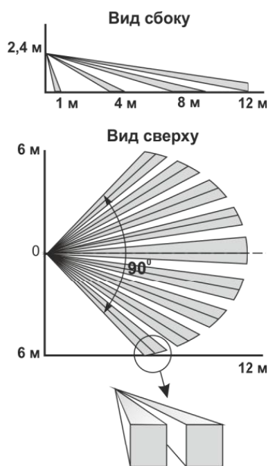
А) СПЕКТРОН-ИО-Объемный-Exi
