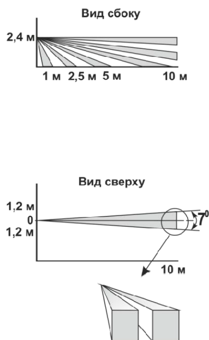
Б) СПЕКТРОН-ИО-Штора-
