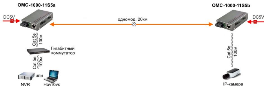
Рис. 4 Схема подключения медиаконвертеров ОМС-1000-11S5a и ОМС-1000-11S5b
