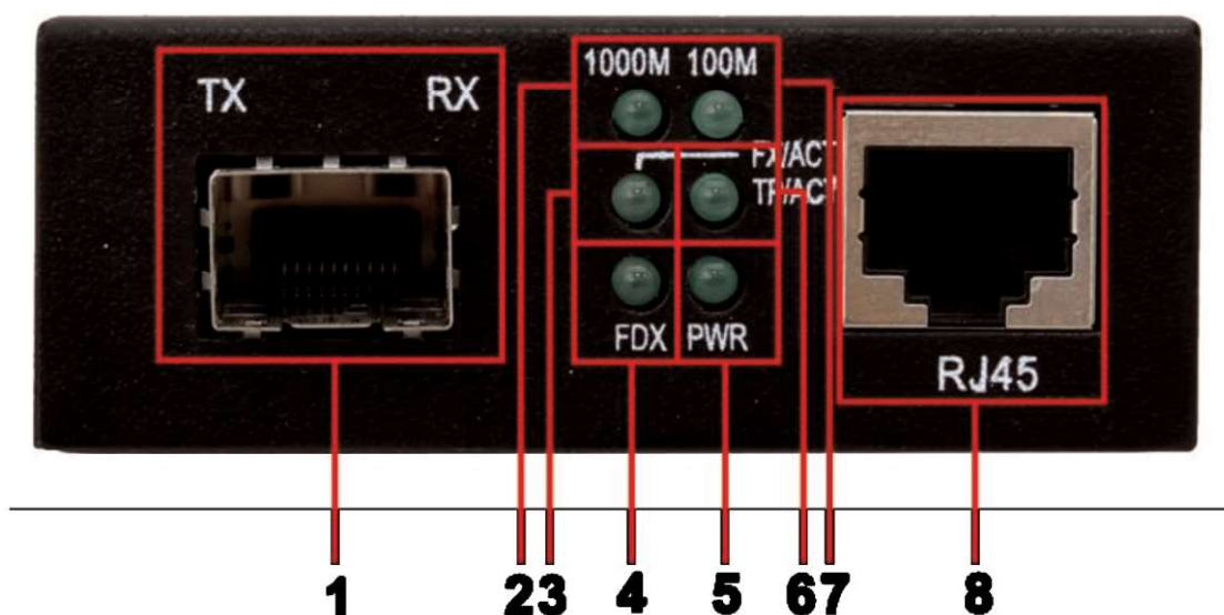
Рис. 3 Медиаконвертер OMC-1000-11X, разъемы и индикаторы на передней панели
