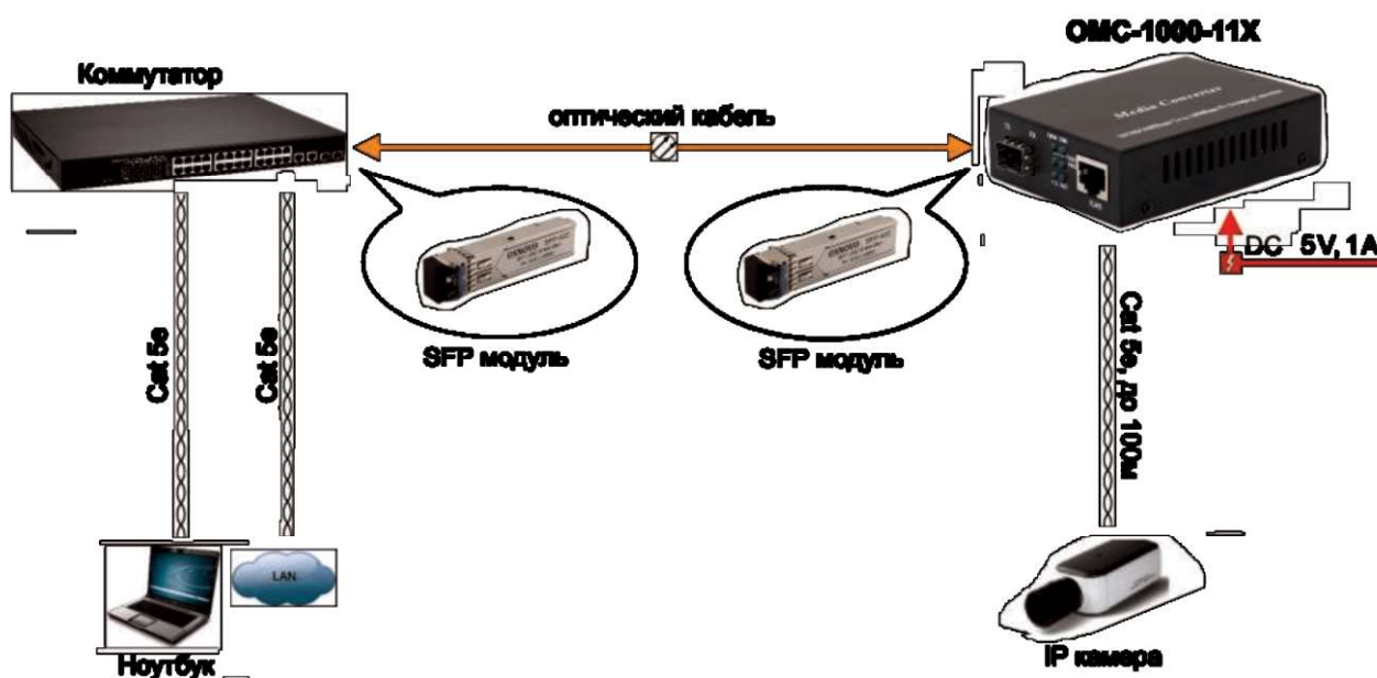
Рис.5 Типовая схема подключения медиаконвертера ОМС-1000-11Х
