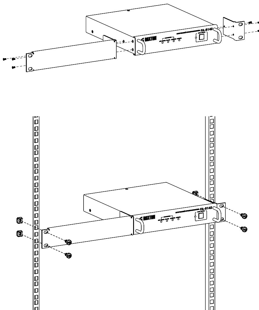
Рисунок Д.2 - Установка изделия в 19" стойку
