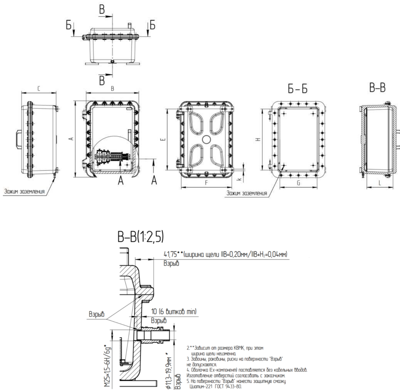
Рис. А1. Общий вид и габаритные размеры коммутационных коробок и Ех-компонентов серии КВМК, моделей: КВМК 1.0 Exd-A-XXX... X, СМД МК 1.0 Exd-A-XXX... X из алюминиевого сплава.
