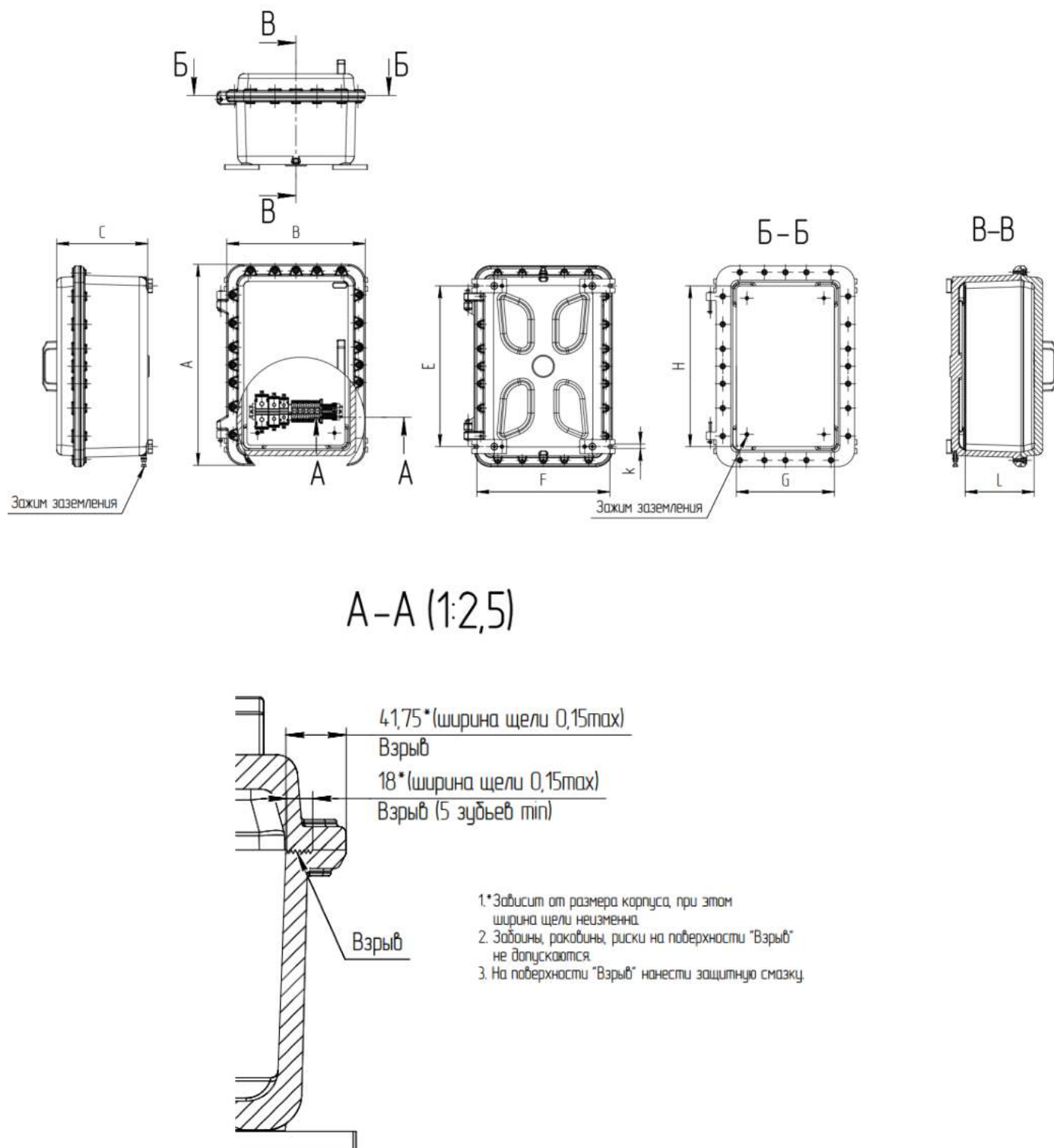
Рис. В1. Общий вид и габаритные размеры коммутационных коробок и Ex-компонентов серии КВМК, моделей: КВМК 1.2 Exd-A-XXX... X, СМД МК 1.2 Exd-A-XXX... X из алюминиевого сплава.
