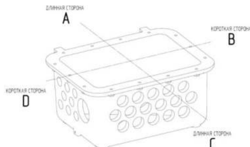
Рис. 1. Схема расположения отверстий под установку кабельных вводов в корпусе серии КВМК, СМД МК, моделей: КВМК 1.0 Exd-A-XXX... X, КВМК 1.0 Exd-H-XXX... X, КВМК 1.2 Exd-A-XXX... X, КВМК 1.2 Exd-H-XXX... X, СМД МК 1.0 Exd-A-XXX... X, СМД МК 1.0 Exd-H-XXX... X, СМД МК 1.2 Exd-A-XXX... X, СМД МК 1.2 Exd-H-XXX... X.
