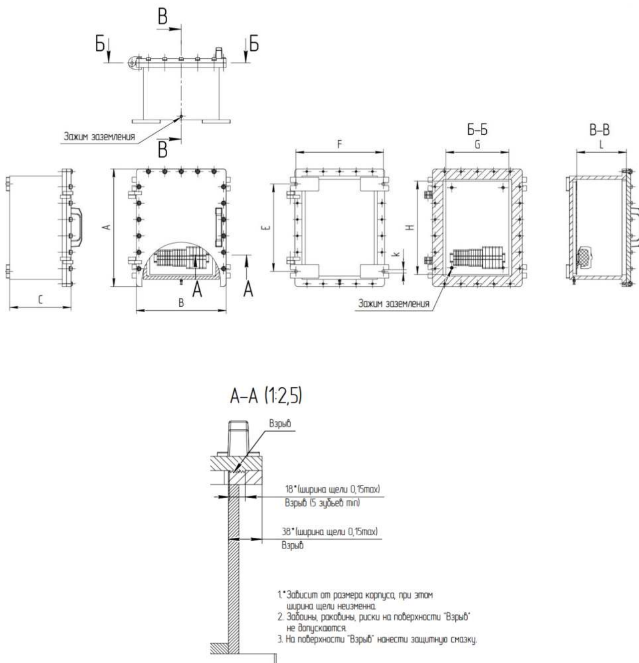
Рис. В2. Общий вид и габаритные размеры коммутационных коробок и Ех-компонентов серии КВМК, моделей: КВМК 1.2 Ехd-Н-XXX... Х, СМД МК 1.2 Ехd-Н-XXX... Х из нержавеющей стали.
