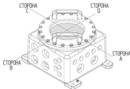
Рис. 2. Схема расположения отверстий под установку кабельных вводов в корпусе серии КВМК, СМД МК, моделей: КВМК 2.1 Exd-A-XXX... X, КВМК 2.1 Exd-H-XXX... X, КВМК 2.3 Exd-A-XXX... X, КВМК 2.3 Exd-H-XXX... X, СМД МК 2.1 Exd-A-XXX... X, СМД МК 2.1 Exd-H-XXX... X, СМД МК 2.3 Exd-A-XXX... X, СМД МК 2.3 Exd-H-XXX... X.
