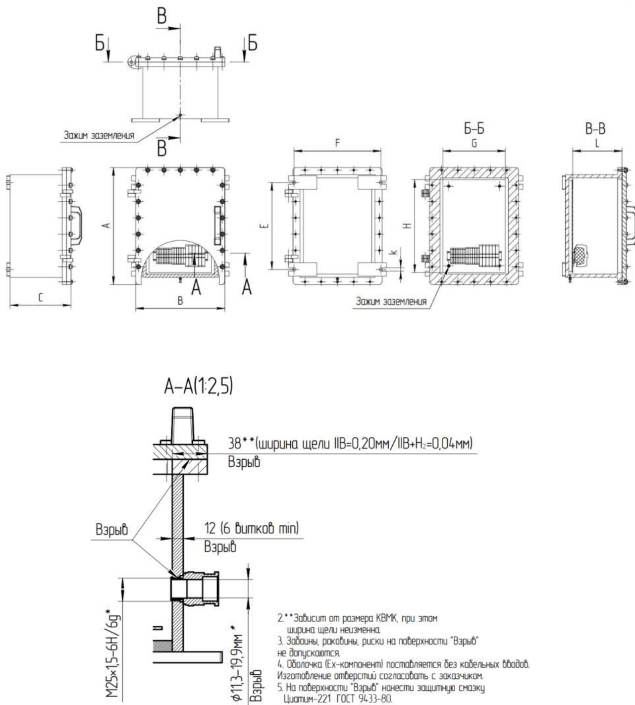
Рис. А2. Общий вид и габаритные размеры коммутационных коробок и Ех-компонентов серии КВМК, моделей: КВМК 1.0 Ехd-Н-XXX... Х, СМД МК 1.0 Ехd-Н-XXX... Х из нержавеющей стали.
