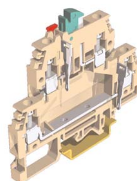
Клеммный зажим DSS.4 с размыкаемым верхним уровнем и перемычками PTC/4 на обоих уровнях
