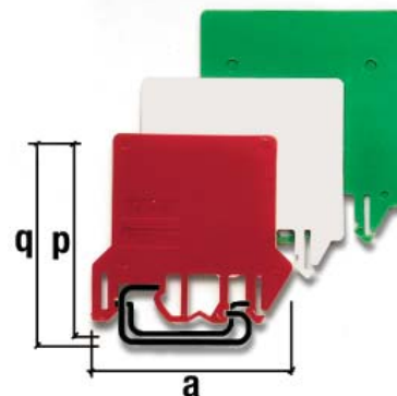
Примечание: размер q больше на 4 мм размера p
