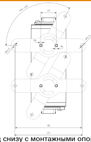
Габаритный чертеж
