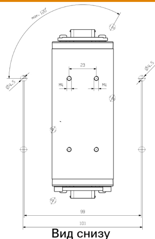
Габаритный чертеж
