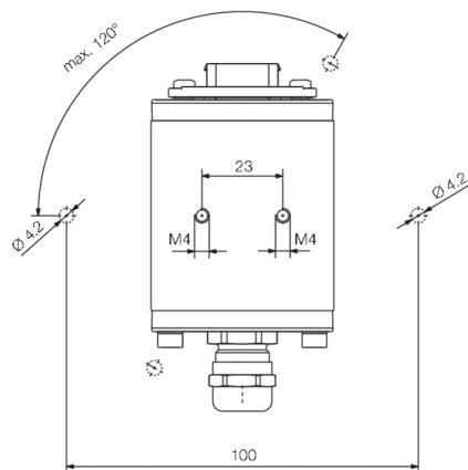
Вид снизу
