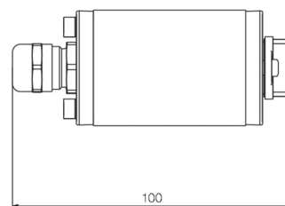
Вид сбоку
