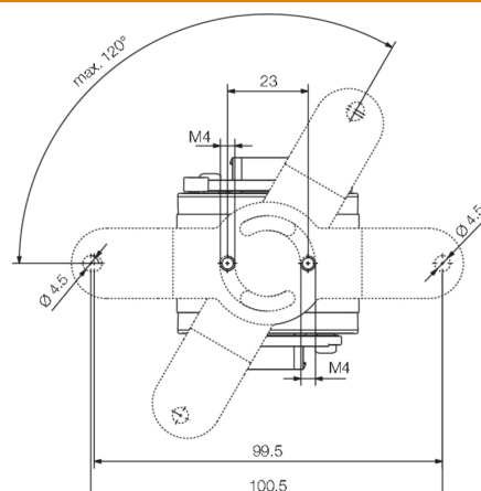
Вид снизу с монтажной опорой
