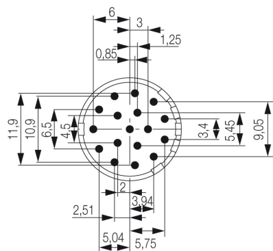
Габаритный чертеж
