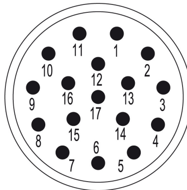
Развод контактов
