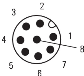
Штекер
