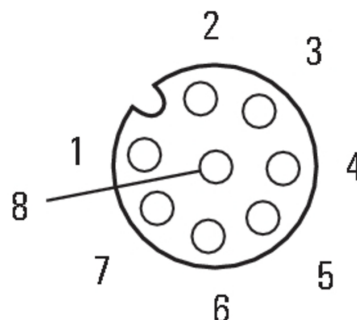
Гнездо
