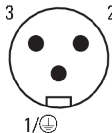
Штекер
