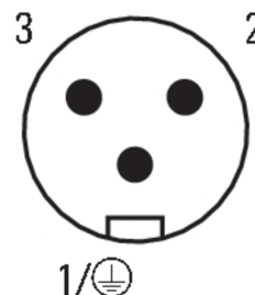
Штекер
