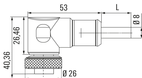
Штекер (угловой)
