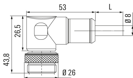
Гнездо (угловое)
