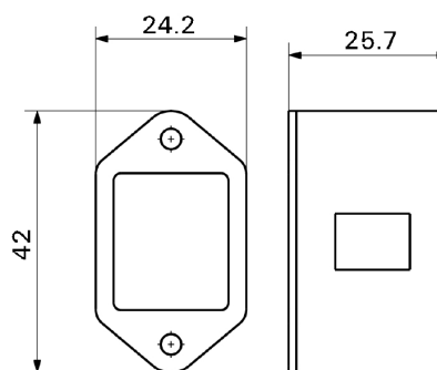
Габаритный чертеж
