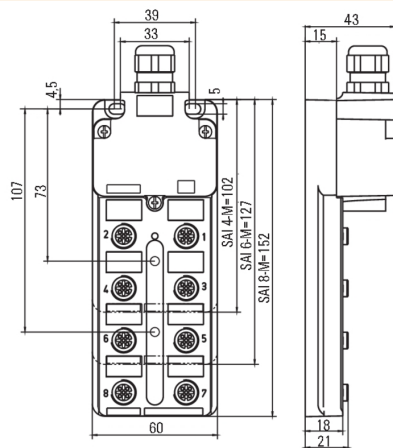
Габаритный чертеж
