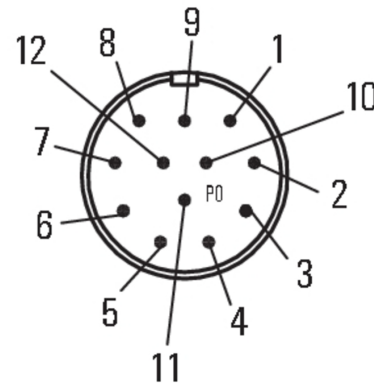
Штекер
