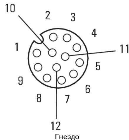
Гнездо (прямое)
