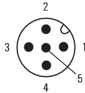
Штифт
