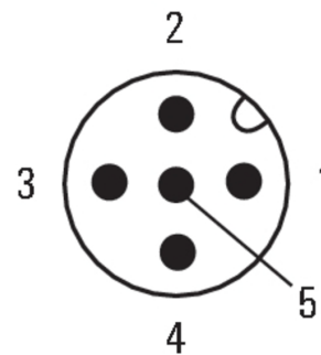
Штифт
