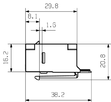
Габаритный чертеж
