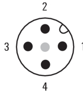
Штекер
