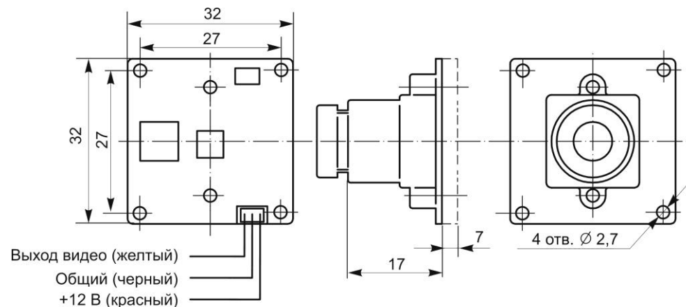
Рис.1. Установочные размеры и схема подключения ТВ камеры.
