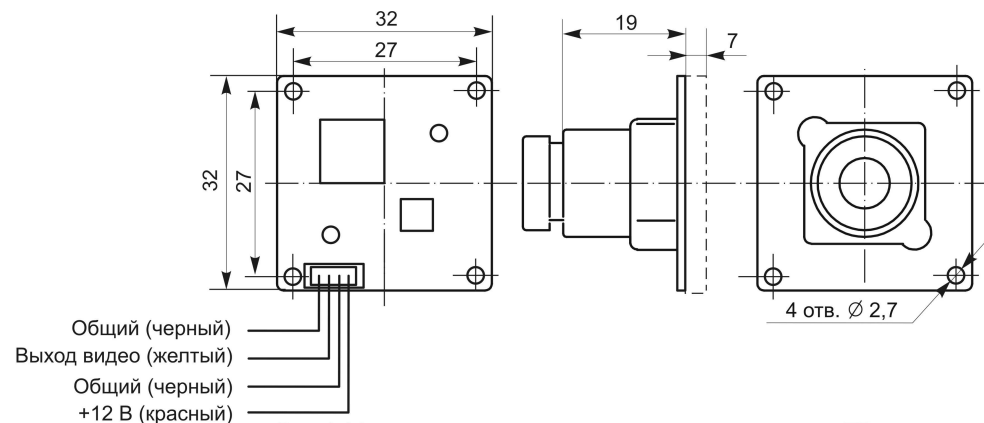
Рис.1. Установочные размеры и схема подключения ТВ камеры.
