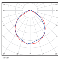
Угол излучения 120°
