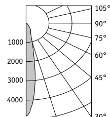
JET/T LED 50 D15
