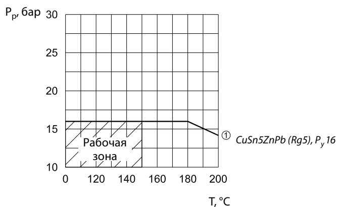
Зависимость рабочего давления от температуры регулируемой среды (в соответствии с EN 1092-3)
