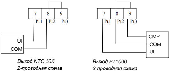
Схема подключения выходов температуры NTC 10K и PT1000
