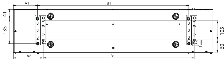
Расположение кронштейнов для установки завесы на шпильки
