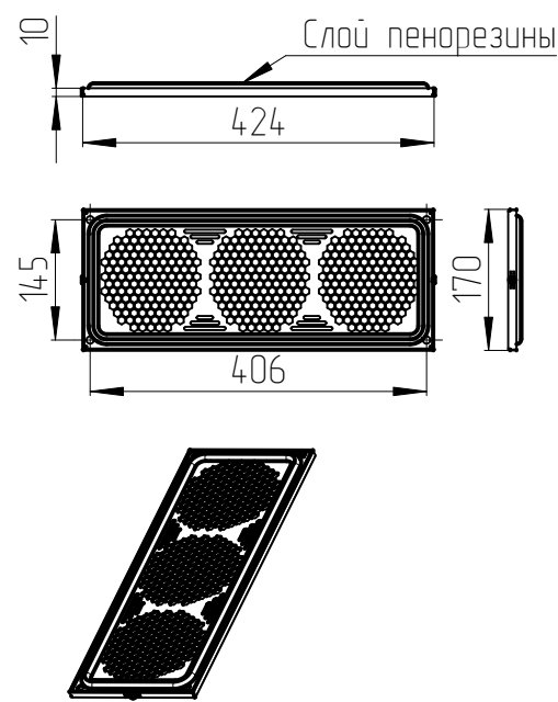
Фильтр МВ-Ф
