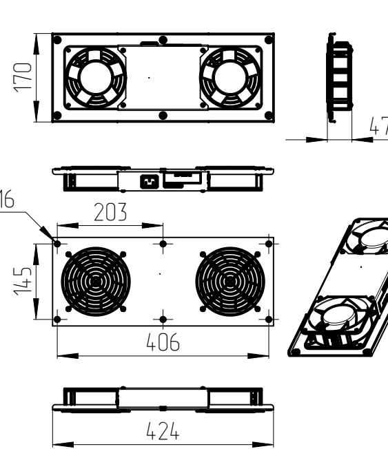
МВ-400-2
