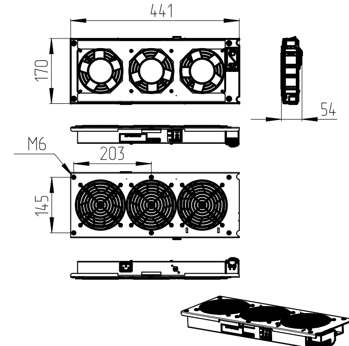
МВ-400-2-3-Т
