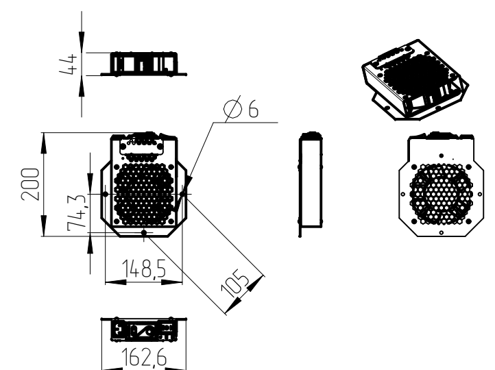
МВ-400-1Т
