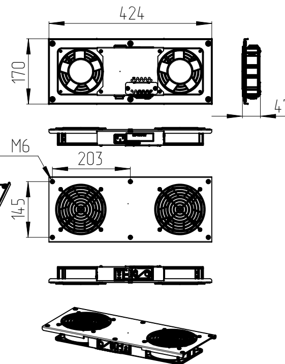
МВ-400-2Т
