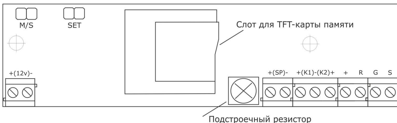
Рисунок 6.2. Внешний вид печатной платы светозвукового табло MP-740R2
