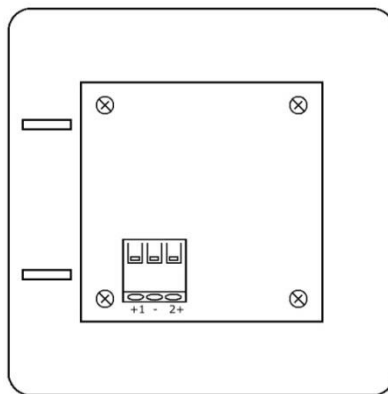
Рисунок 6.1. Внешний вид платы кнопки вызова MP-421D1
