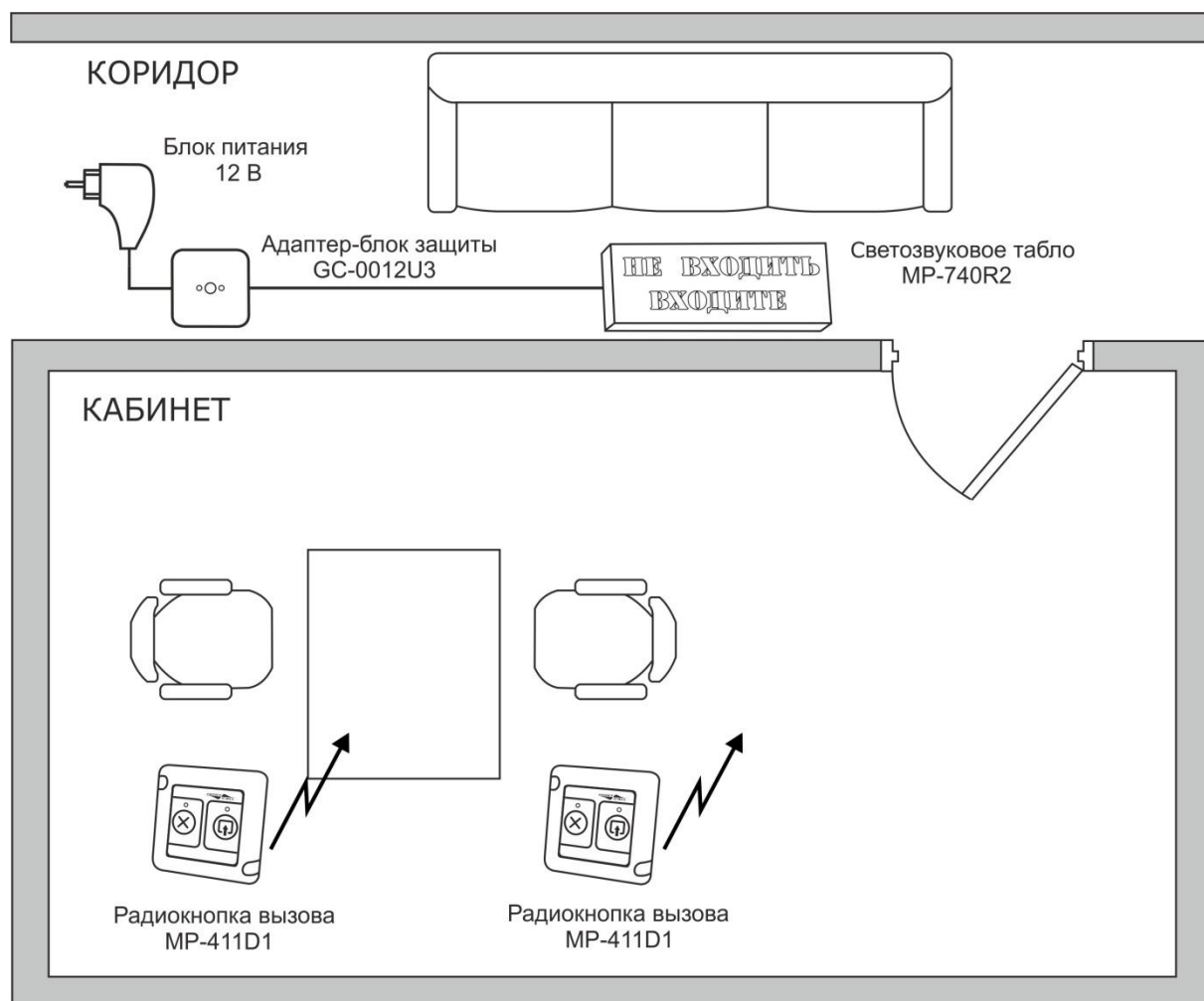
Рисунок 2.2. Структурная схема комплекта вызова MP-911W2
