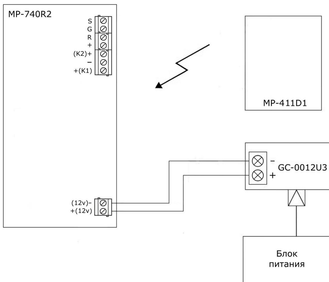
Рисунок 7.5. Схема соединений комплекта вызова MP-911W2
