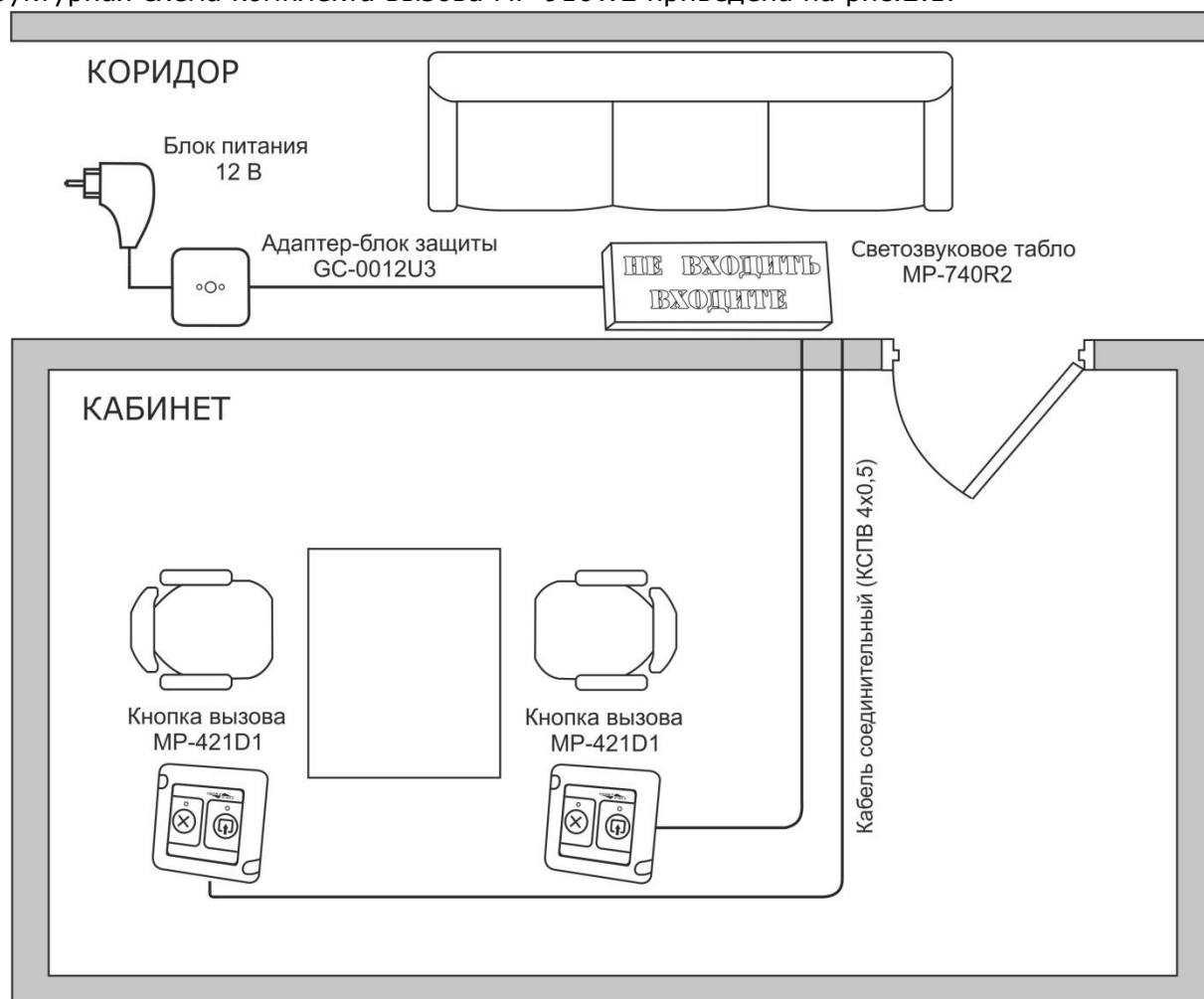
Рисунок 2.1. Структурная схема комплекта вызова MP-910W2
