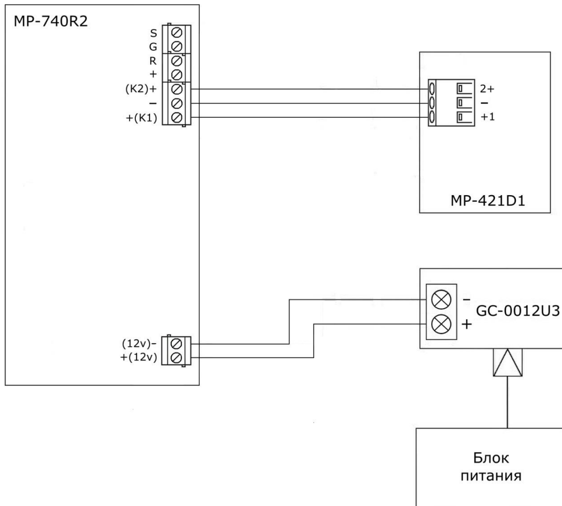
Рисунок 6.4. Схема соединений комплекта вызова MP-910W2
