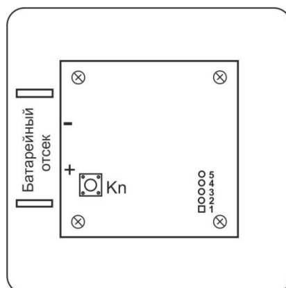
Рисунок 7.1. Внешний вид платы радиокнопки вызова MP-411D1
