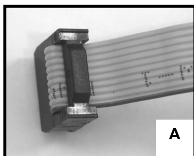
Рисунок 6. Внешний вид кабеля соединительного CB-MR – X.X
