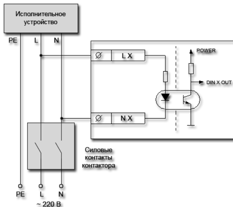
Рис. 26 Пример применения для контроля наличия питающей сети исполнительного устройства
