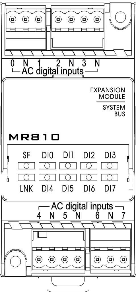
Рис. 23 Внешний вид MR – 0810-0х-х
