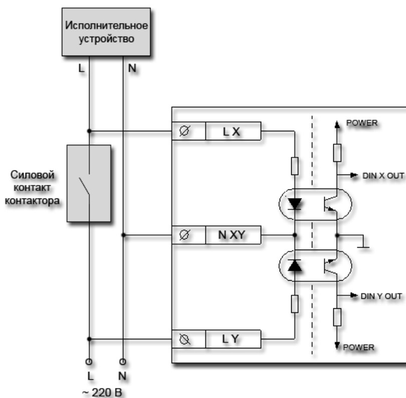
Рис. 27 Пример применения для контроля наличия внешней питающей сети и срабатывания контактов контактора (идеально для клемм 1-3, 12-14)
